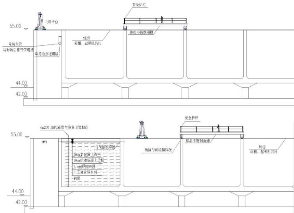
图 4-3 吊装作业示意图
