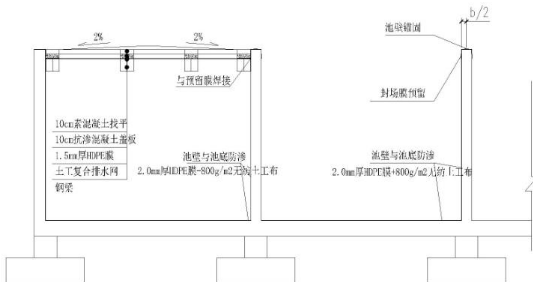
图 4-5 封场结构示意图
