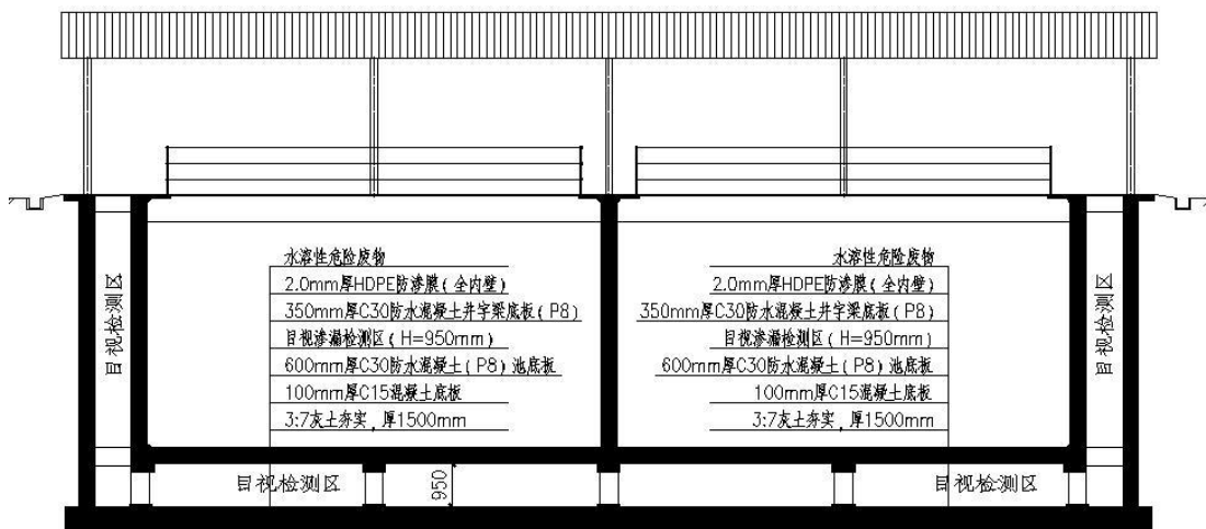
图 4-1 填埋仓单元设计图
