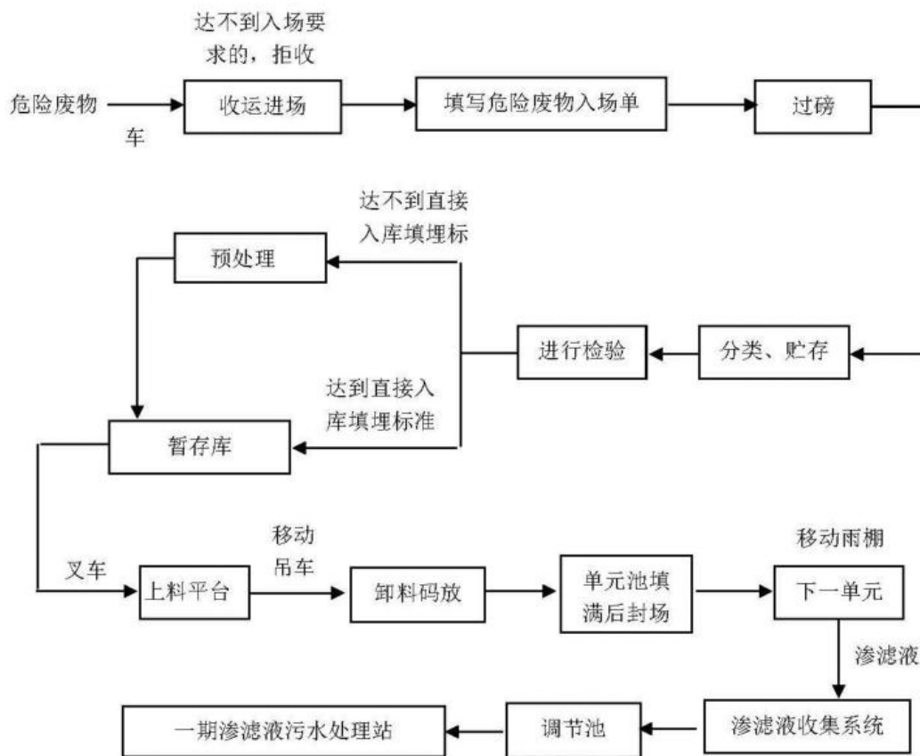
图 3-1 总体工艺流程流程图
