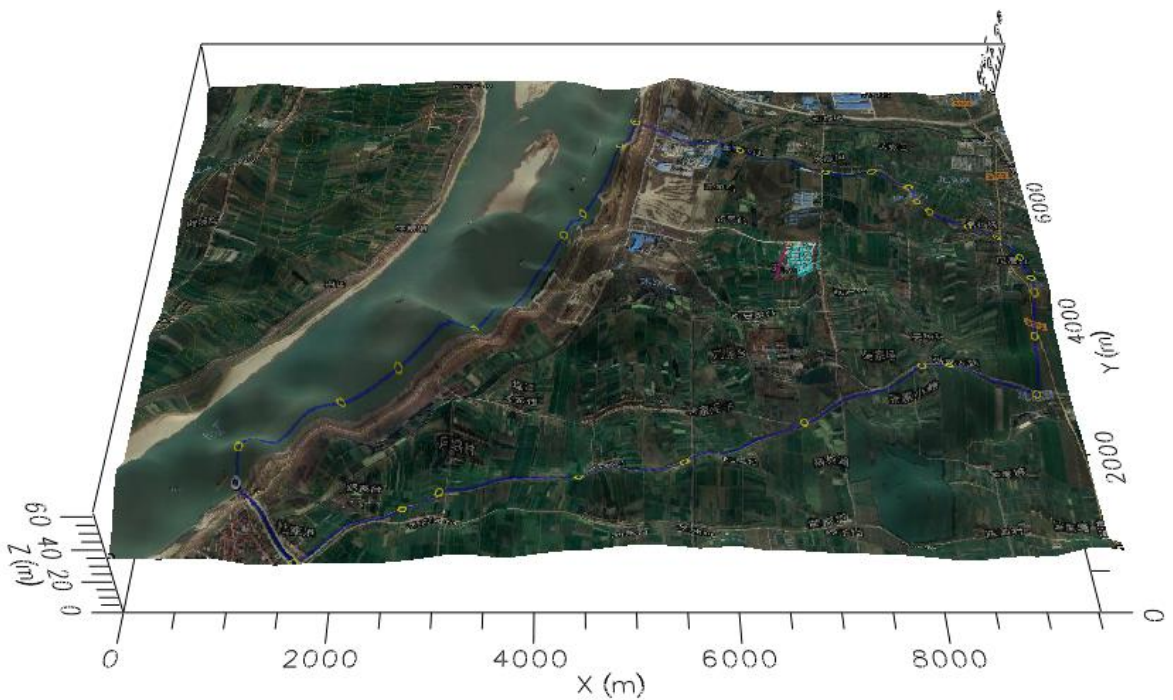
模拟区高程三维图
