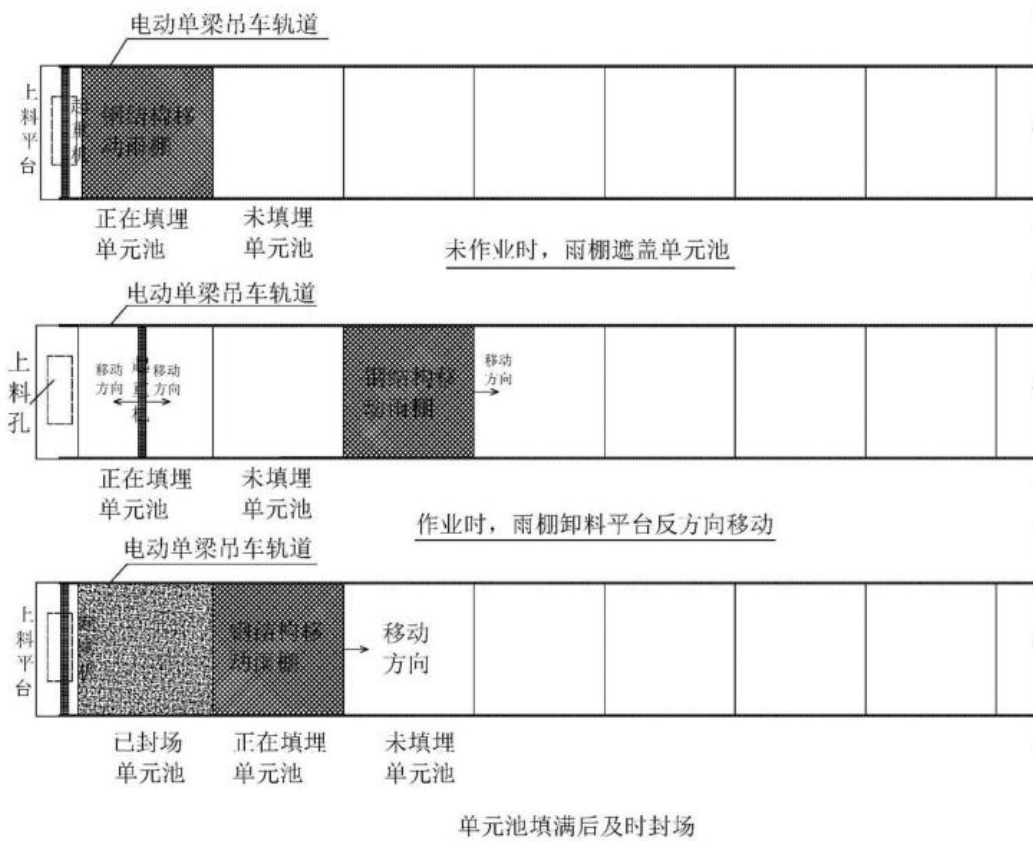
图 4-4 填埋作业流程示意图
