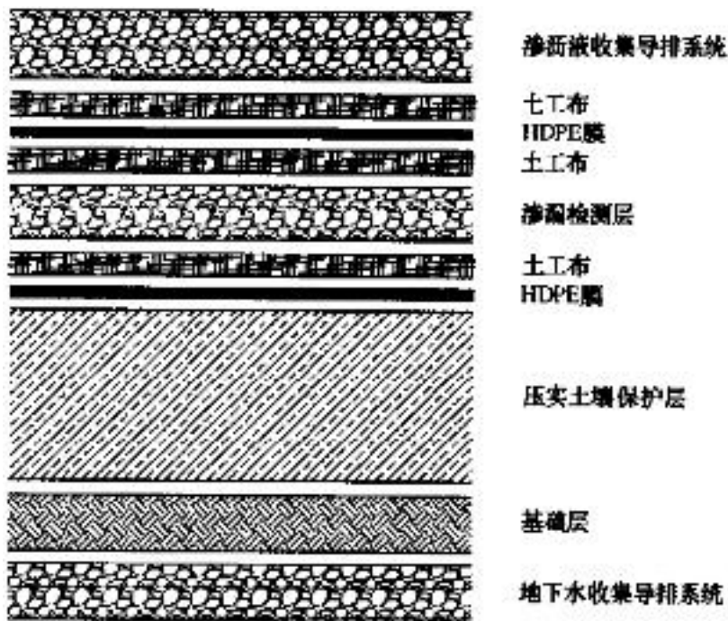
双层防渗结构示意图
