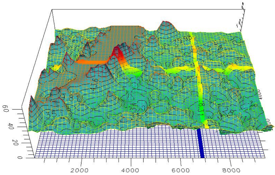
模拟区高程三维图(Z轴 50 倍拉伸)
