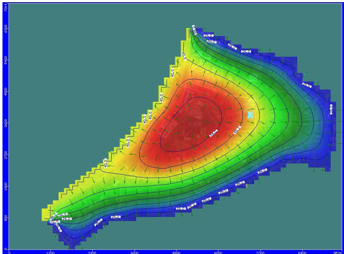
本项目初始渗流场
