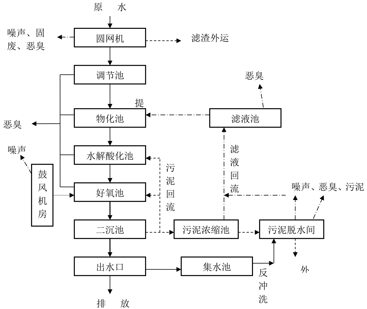
图 6-8 污水处理厂工艺流程
