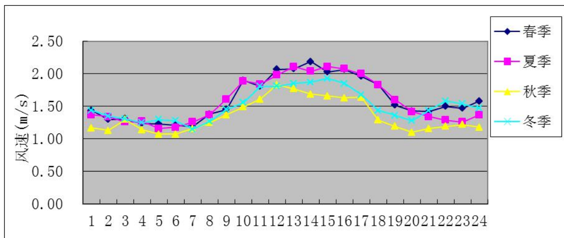
图 6-3 季小时平均风速日变化曲线图
